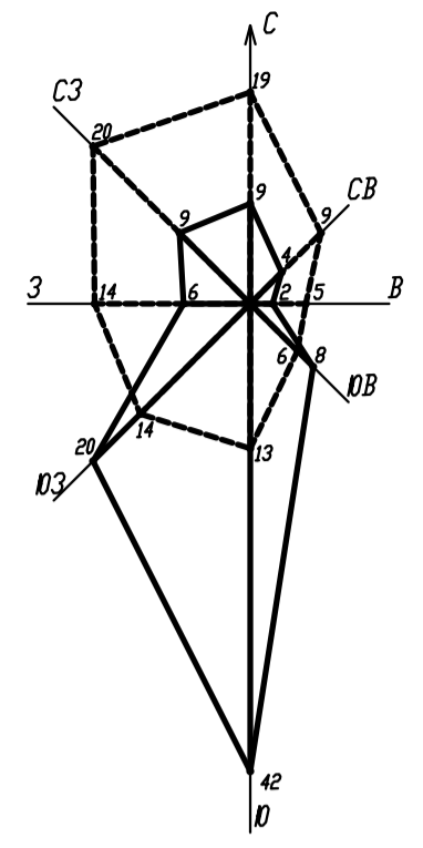
Роза ветров по повторяемости направления ветра, % — за январь — за июль
